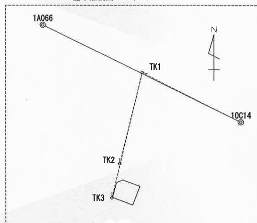
基準点網図 S=1/2000
