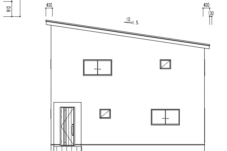
西側 立面図 S:1/100
